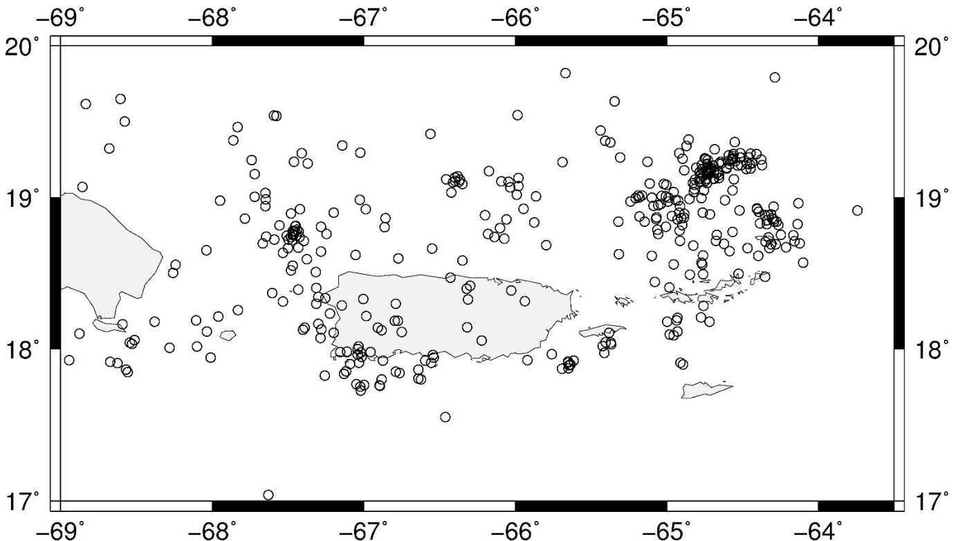
Figura 1. Mapa epicentral de los sismos localizados por la RSPR para el mes de agosto de 2016 (RSPR-UPRM).
